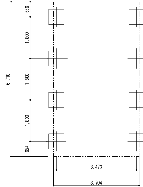
■ 基礎配置図
